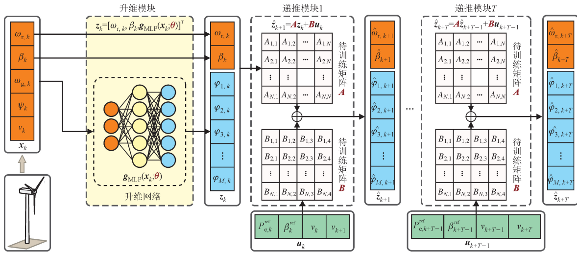
图 1 状态空间映射神经网络 Fig. 1 State-space mapping neural network
