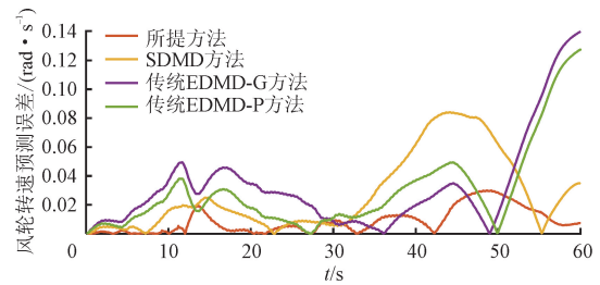
(b) 风轮转速预测误差
