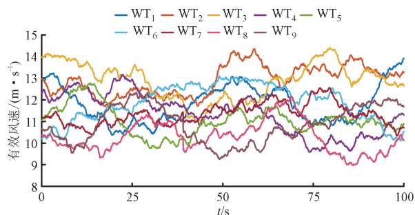
图 6 风电机组的有效风速
