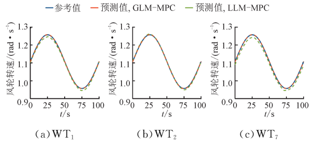
图 8 控制场景 1 下 WT 1 、WT 4 和 WT 7 的风轮转速曲线
