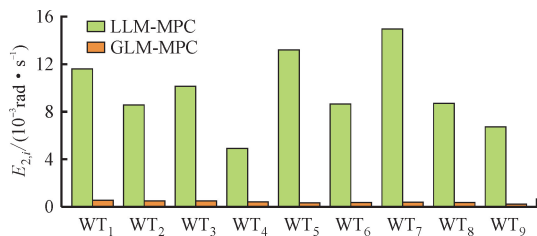
图9 各个风电机组的转速越限程度
