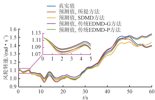
(a) 风轮转速预测结果
