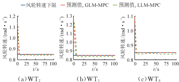
图10 控制场景2下 WT 2 、WT 5 和 WT 8 的风轮转速曲线
