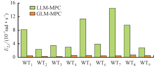
图 7 各个风电机组的转速跟踪误差
